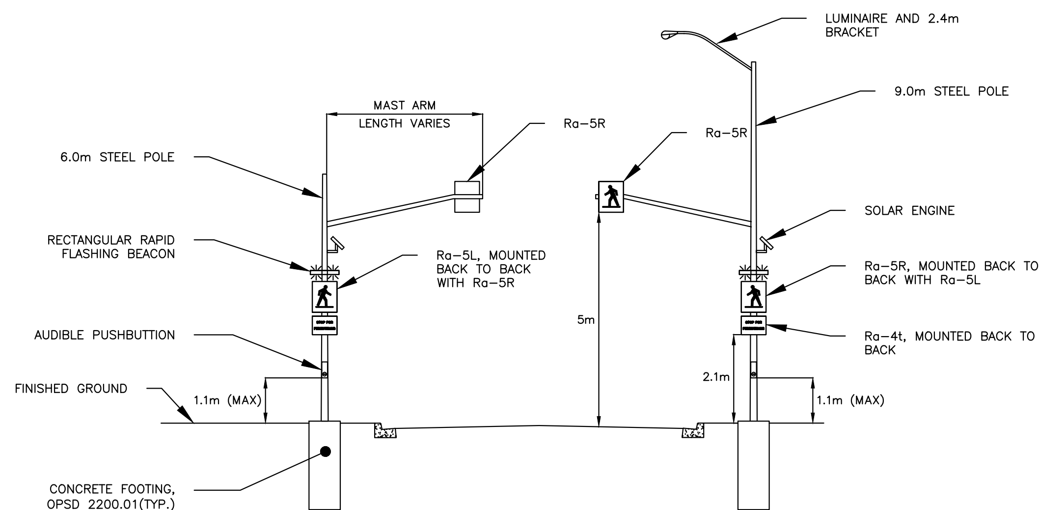
POLE INSTALLATION TYPE B N.T.S.
